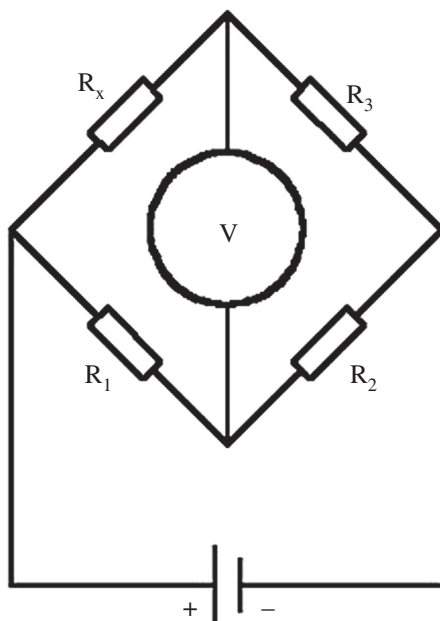
Fig. 3: Schema van de in 1843 door Charles Wheatstone bedachte schakeling.
